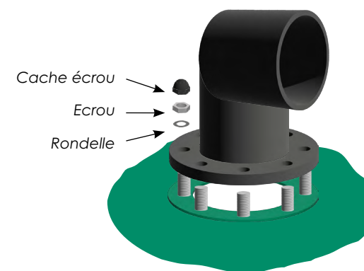
Trop-plein/Dégazeur
