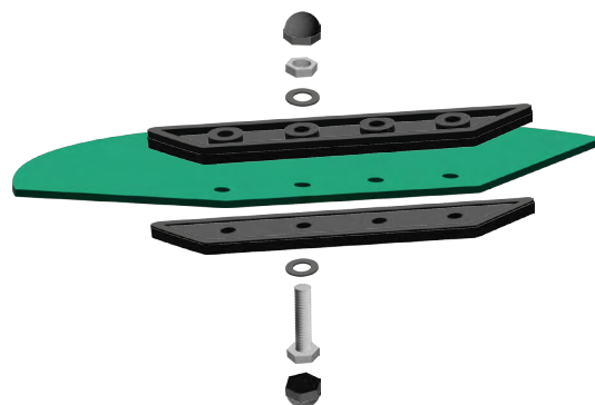
Plaquette de renfort d'angle
